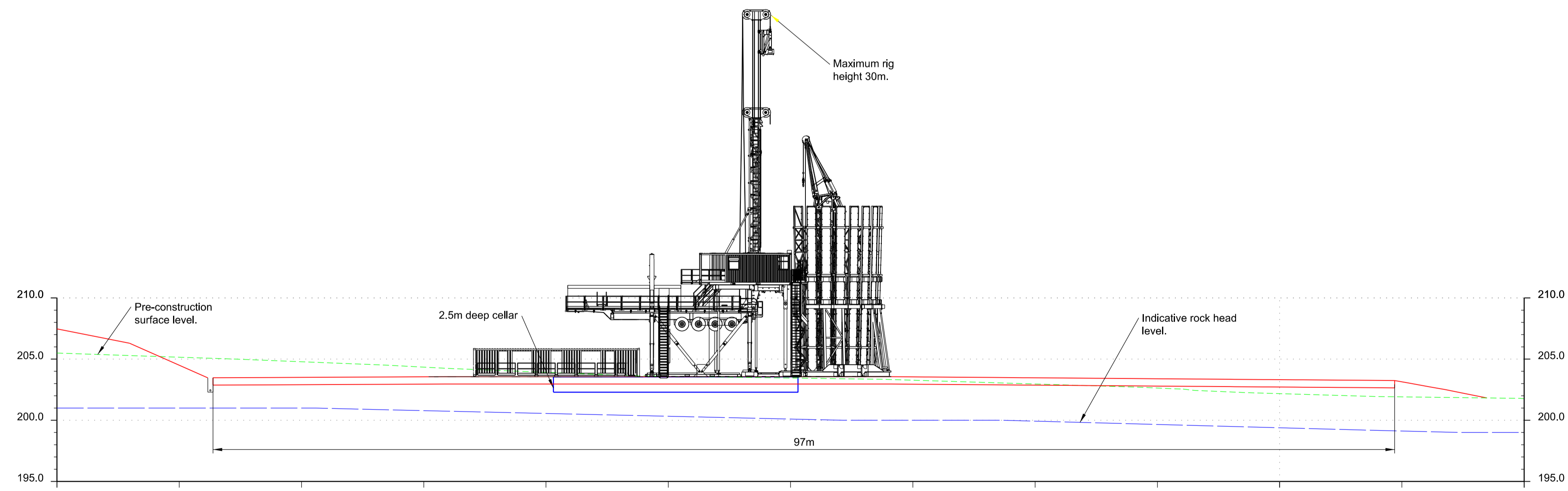
Section A-A Scale H 1:250 V 1:250
