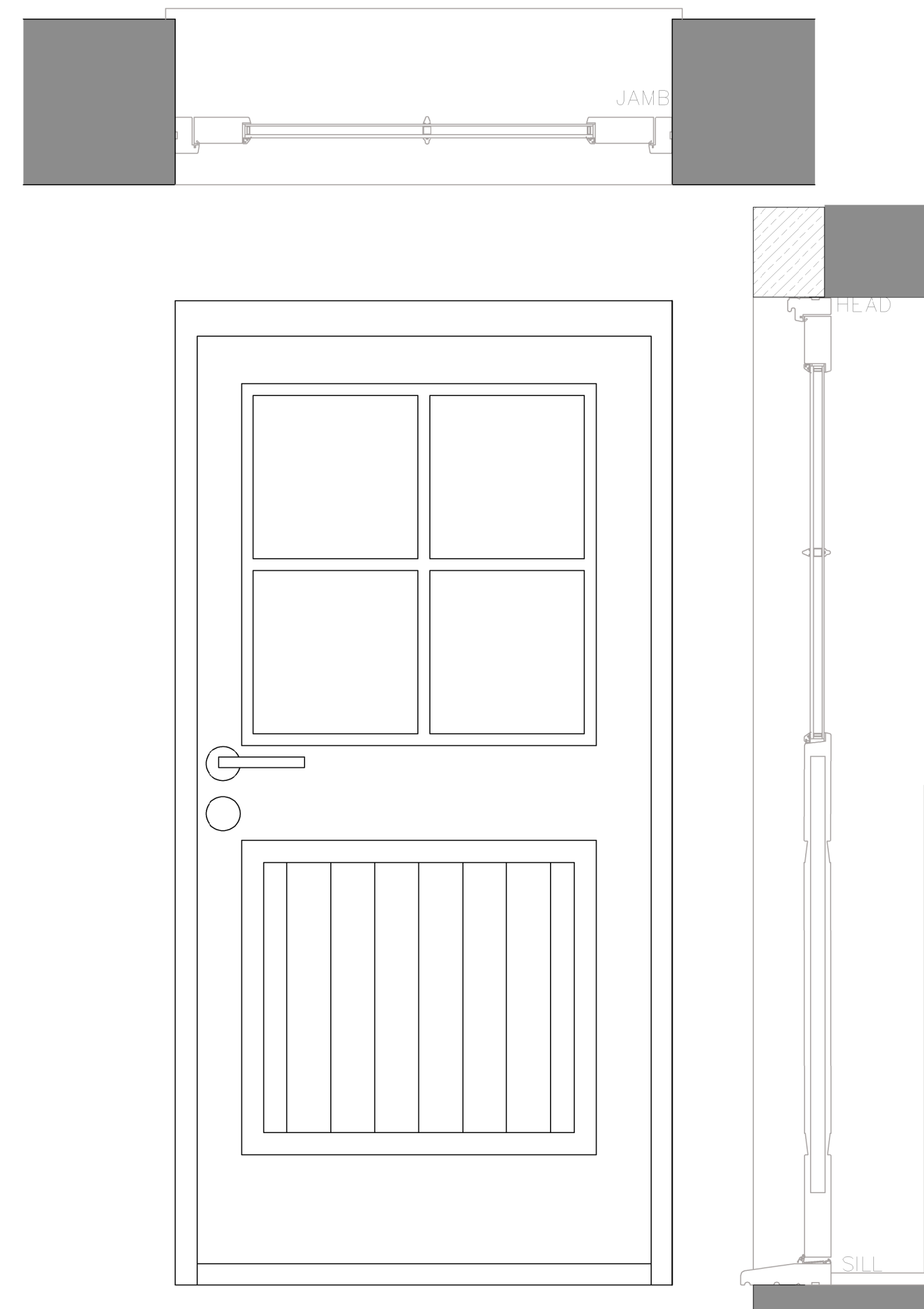
External Door Details - 1:10
