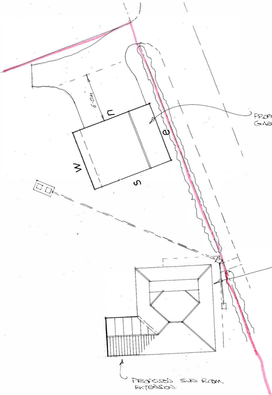
Site Layout 1:200
